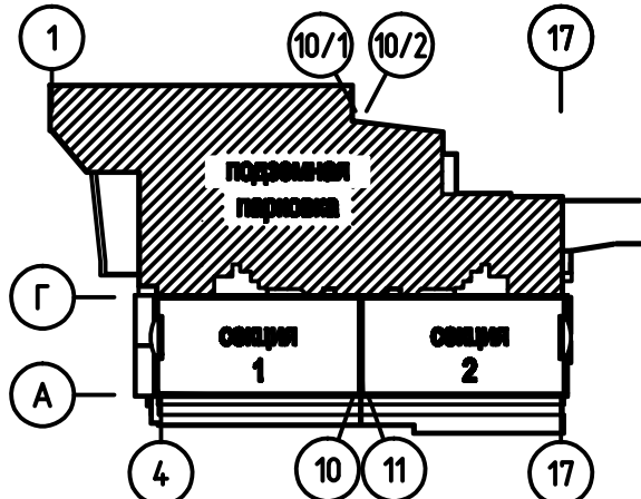
КОМПОНОВочная СХЕМА
